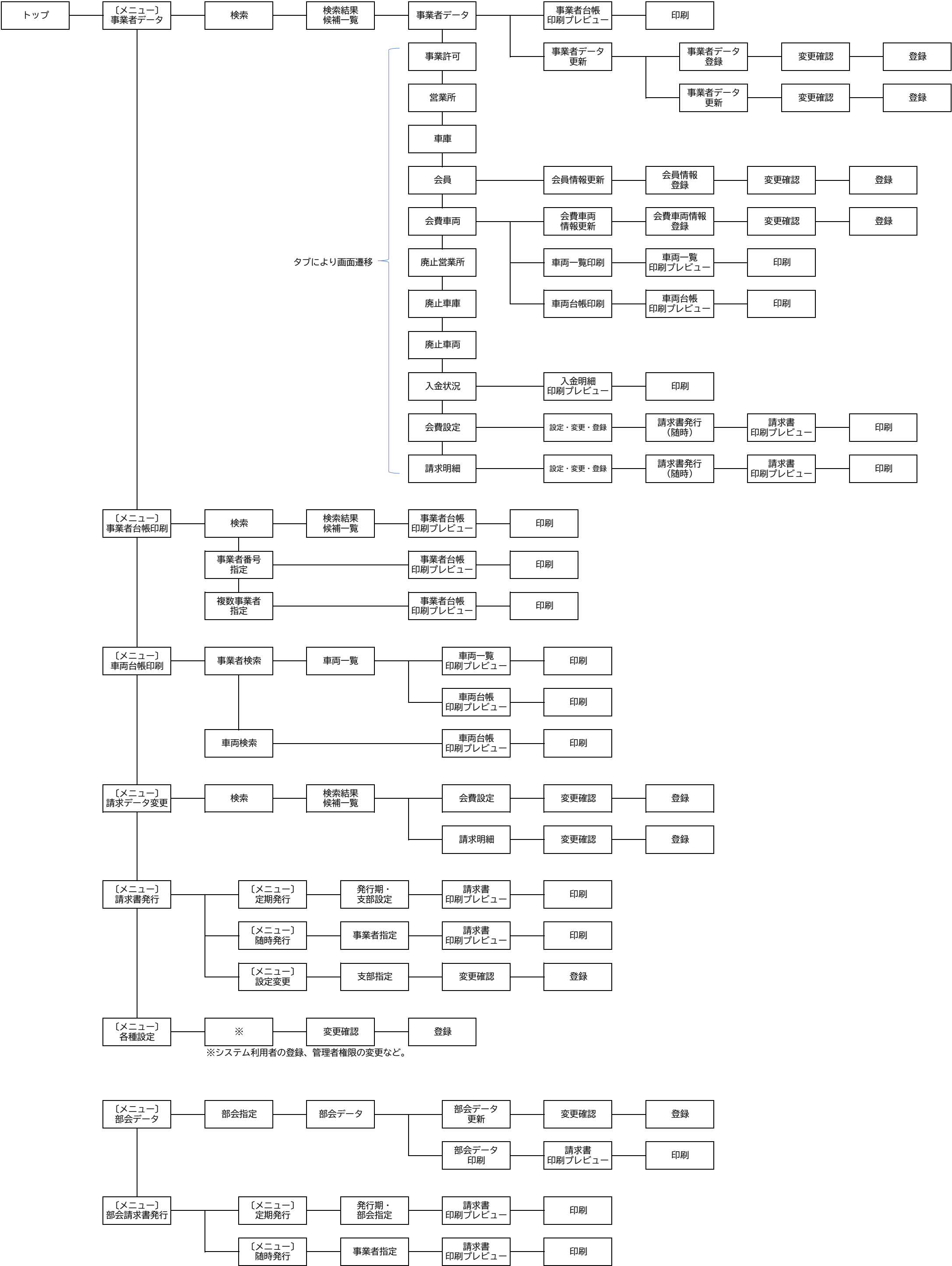
【参考】システム画面遷移図（案） 現時点で想定される大まかなメニューおよび画面遷移です。
