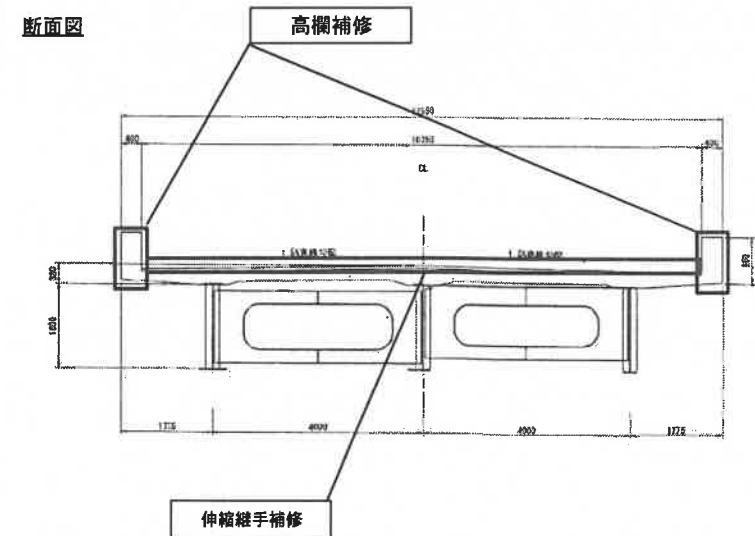
断面図
