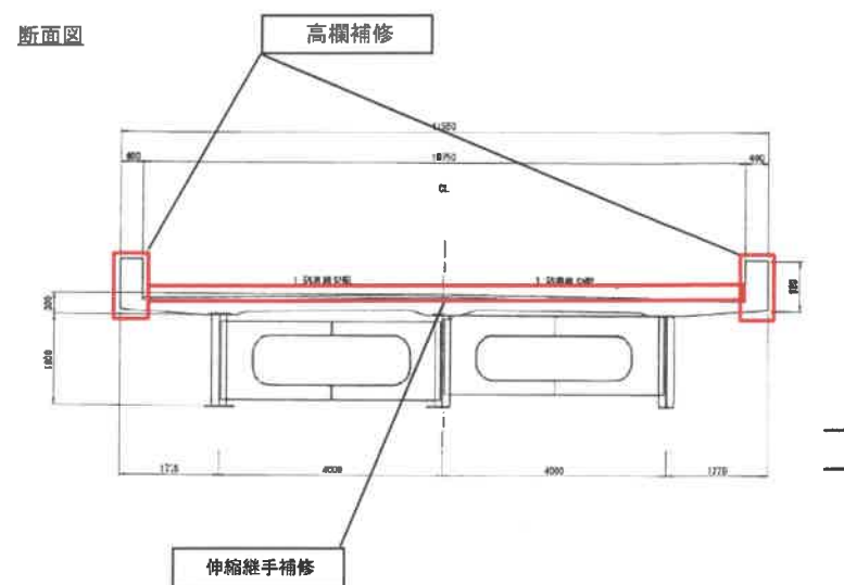
断面図
