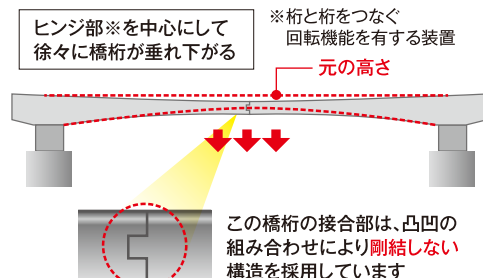
橋桁の中央付近が設計時の想定よりも大きく沈下
