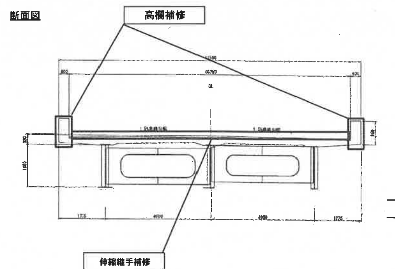
断面図
