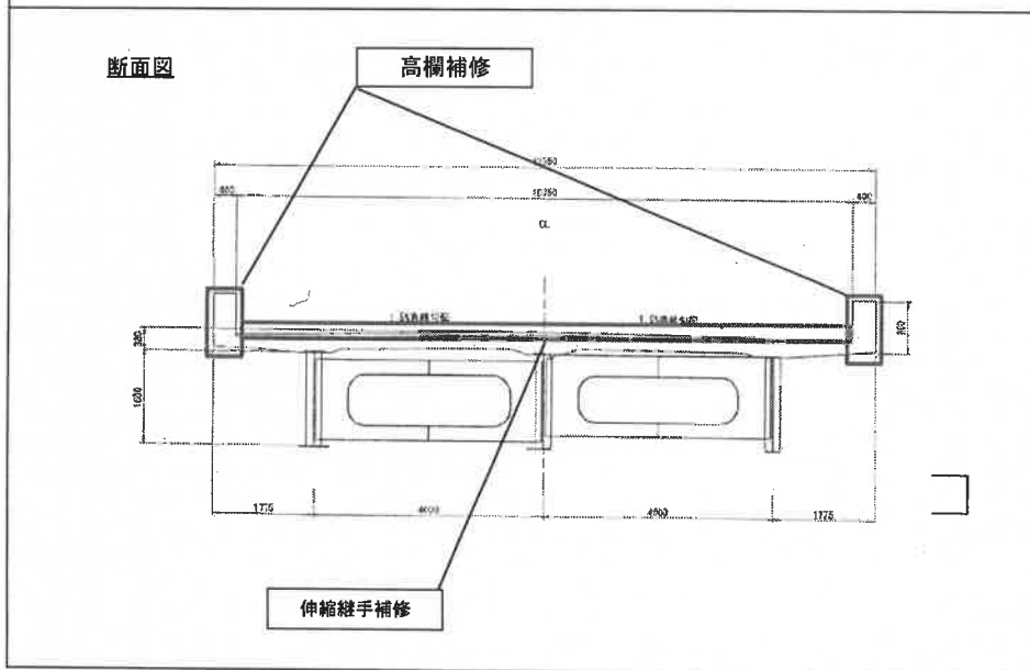
断面図
